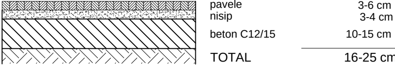
Trotuar pavele
