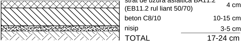
Trotuar asfalt
