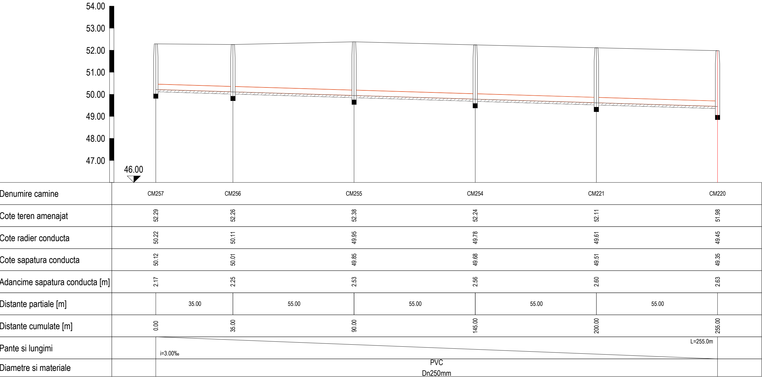
PROFIL LONGITUDINAL REȚEA CANALIZARE MENAJERA PE STRADA NR.18 Tronson CM257 - CM220
