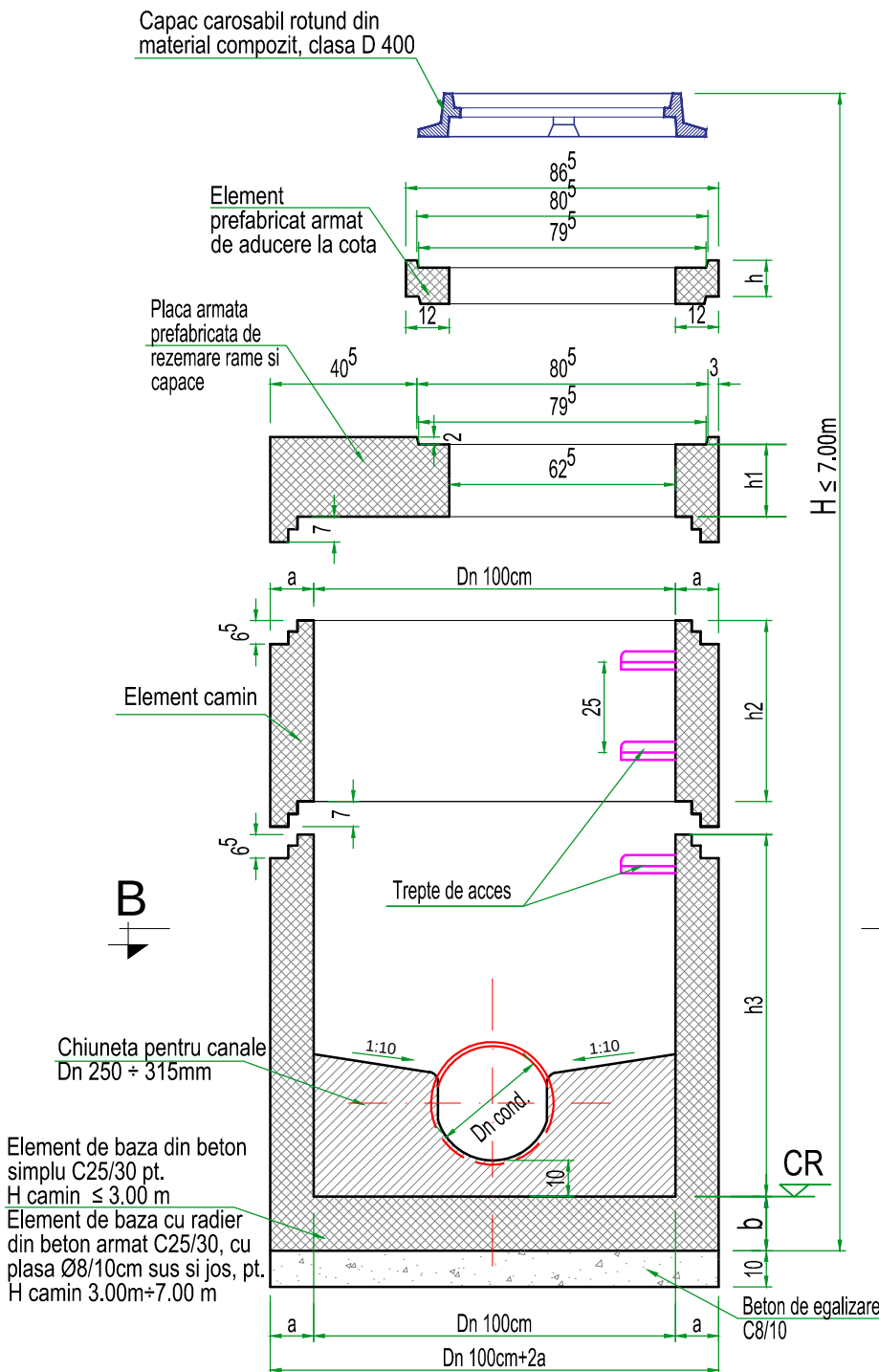
Sectiunea A-A
