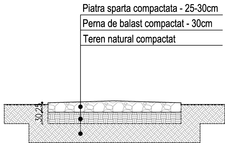
SECȚIUNE TRANSVERSALA D-D - PLATFORMA ACCES
