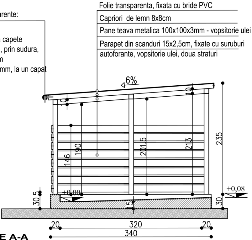
SECTIUNE A-A
