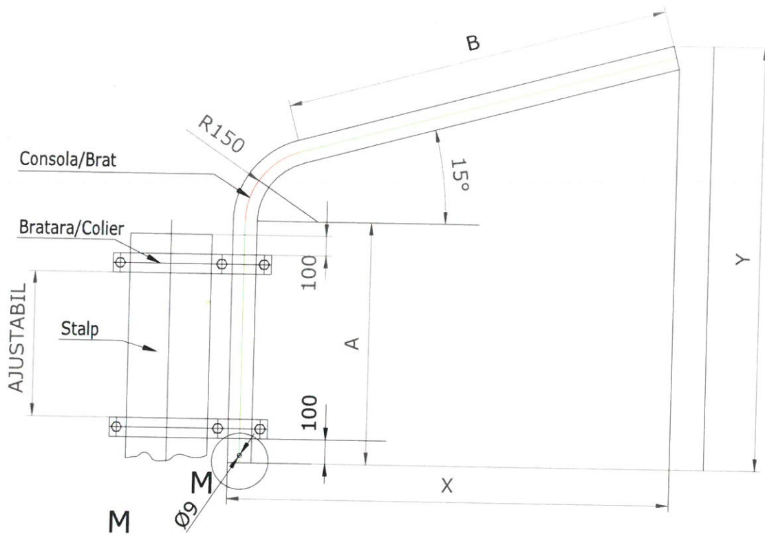
Scara 1:2
